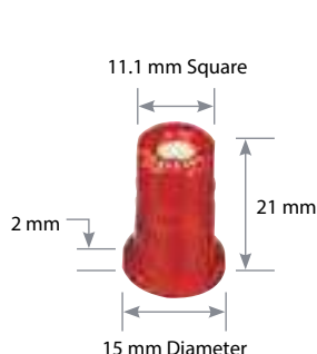
TXA ConeJet
