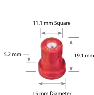
TXB ConeJet
